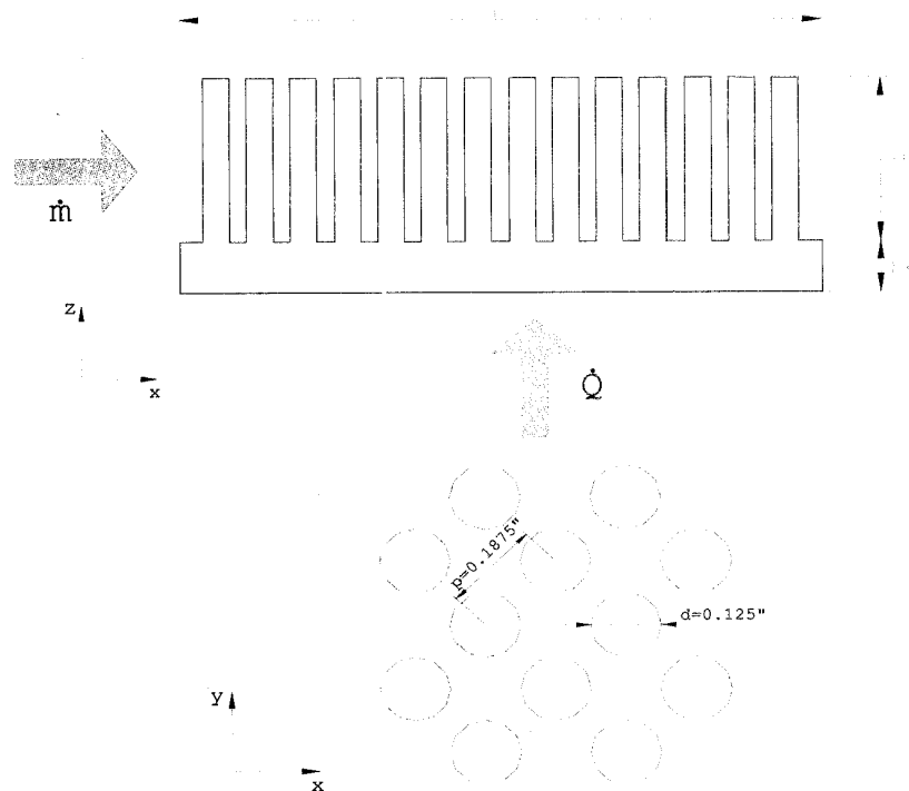
Sl. 1. Eksperimentalna testna proga
