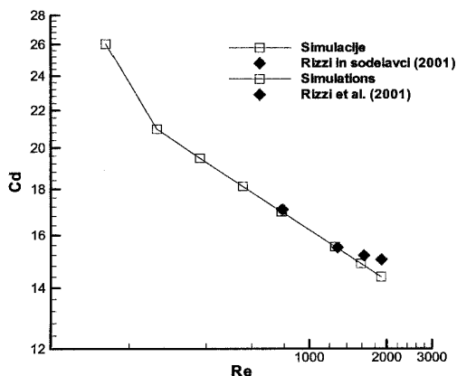
Sl. 4. Koeficient upora celotne sekcije kot funkcija Reynoldsovega števila Fig. 4. Whole-section drag coefficient as a function of Reynolds number
