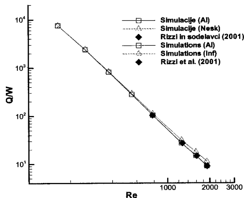
Sl. 6. Toplotna učinkovitost hladilnika v odvisnosti od Reynoldsovega števila Fig. 6. Heat-sink effectiveness as a function of Reynolds number
