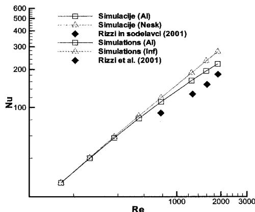
Sl. 5. Nusseltovo število celotne sekcije kot funkcija Reynoldsovega števila Fig. 5. Whole-section Nusselt number as a function of Reynolds number
